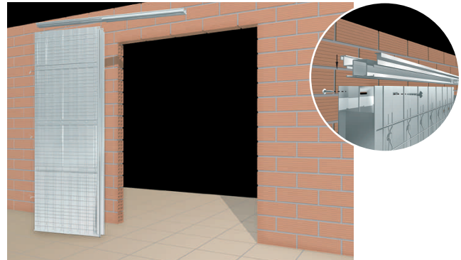
2. Colocación del perfil superior en la estructura metálica. Fitting of upper track to metal frame. Pose du profilé supérieur sur la structure métallique.
